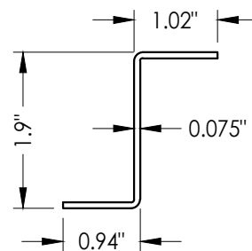
87 Z ASTRAGAL
